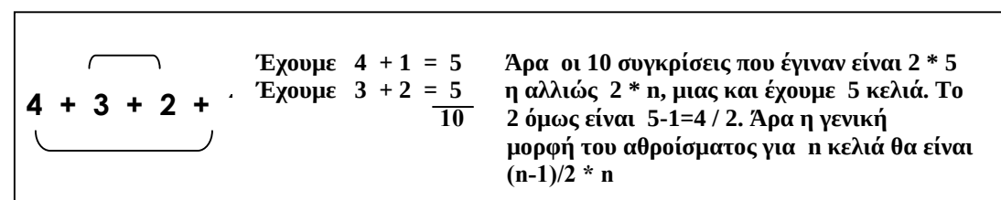
Σχήμα 5: Υπολογισμός του αθροίσματος
