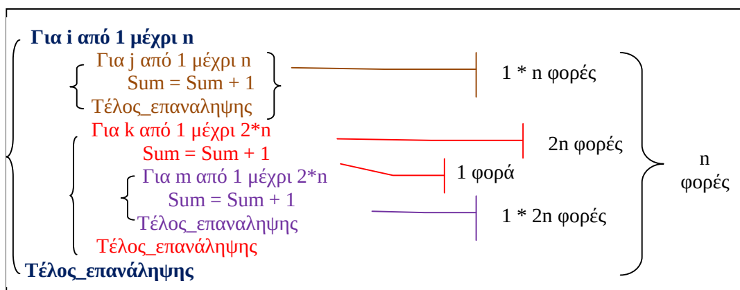
Σχήμα 2: Παράδειγμα Πολυπλοκότητας
