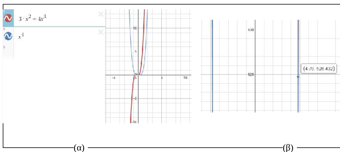
Σχήμα 3: Γραφικές παραστάσεις των f(n) , g(n)
